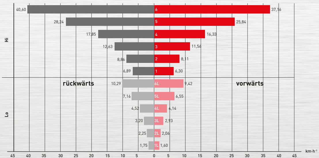
12/12 Wendegetriebe (Bereifung hinten 18,4 R34)
